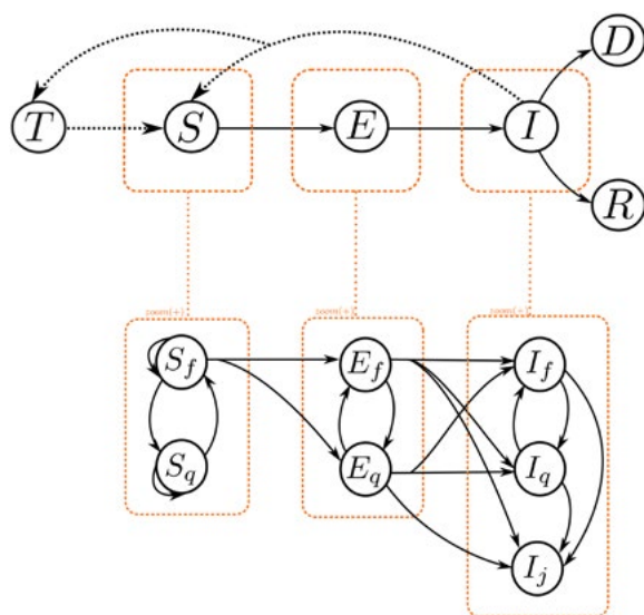
Figura 1. Modelo matemático utilizado. Plan Cosecha Cafetera. Universidad EAFIT proyecto MathCOVID — https://journals.plos.org/plosone/article?id=101371/journal.pone0275546
